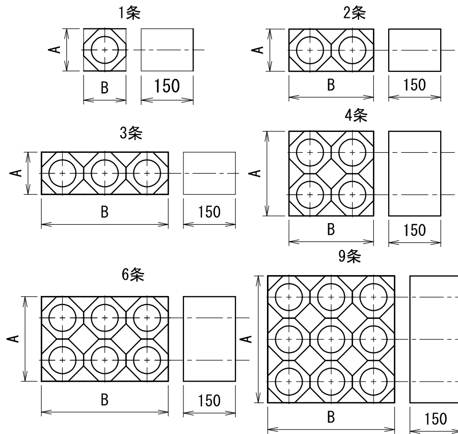
製品仕様図
